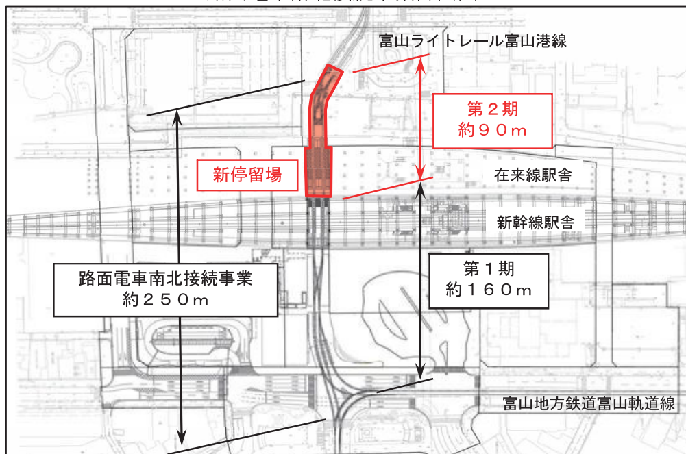
路面電車南北接続事業計画図
