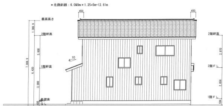
西側立面図 S:1/100
