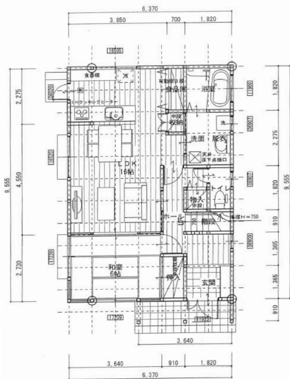
1階平面図
