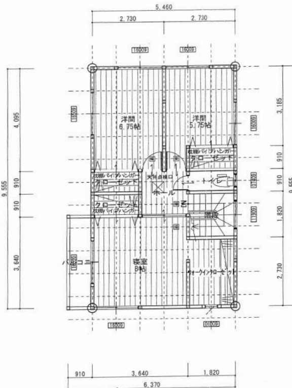
2階平面図
