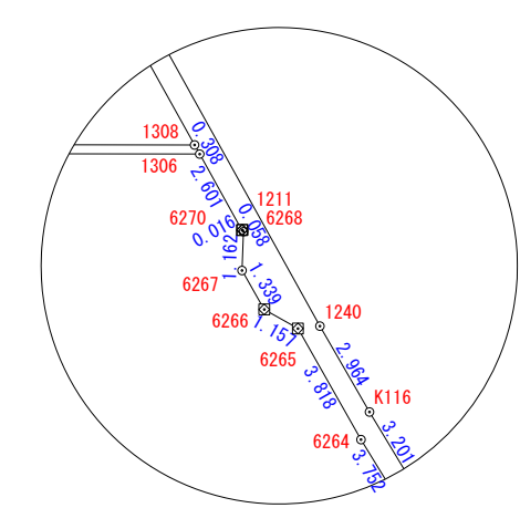
拡大図 1/250
