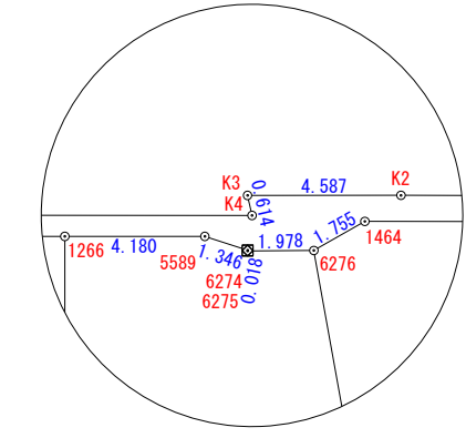
拡大図 1/250
