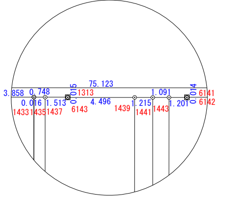
拡大図 1/250
