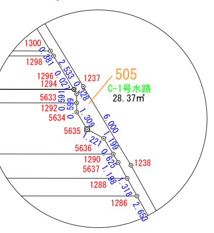
拡大図 1/250
