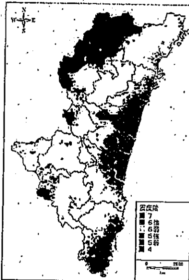
震度分布
