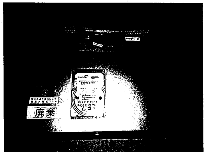
破壊後 No.5 NEC ノートパソコン PC-NS750DAG
