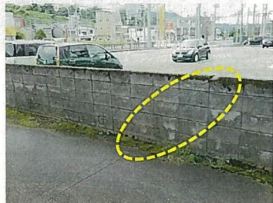
ひび割れ2.6m
