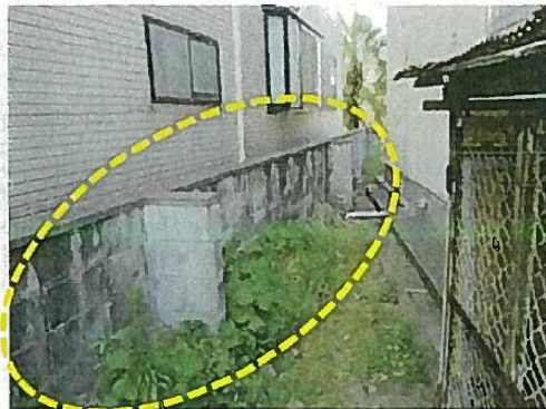
塀の高さ113cm、長さ44m、控壁の長さ40cm、控壁の間隔 最長7.7m
