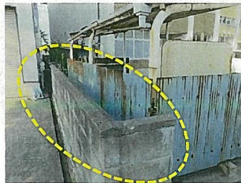
塀の高さ113cm、長さ44m、控壁の長さ40cm、控壁の間隔 最長7.7m
