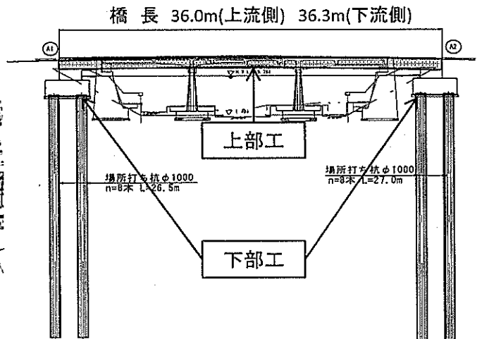
側面図
