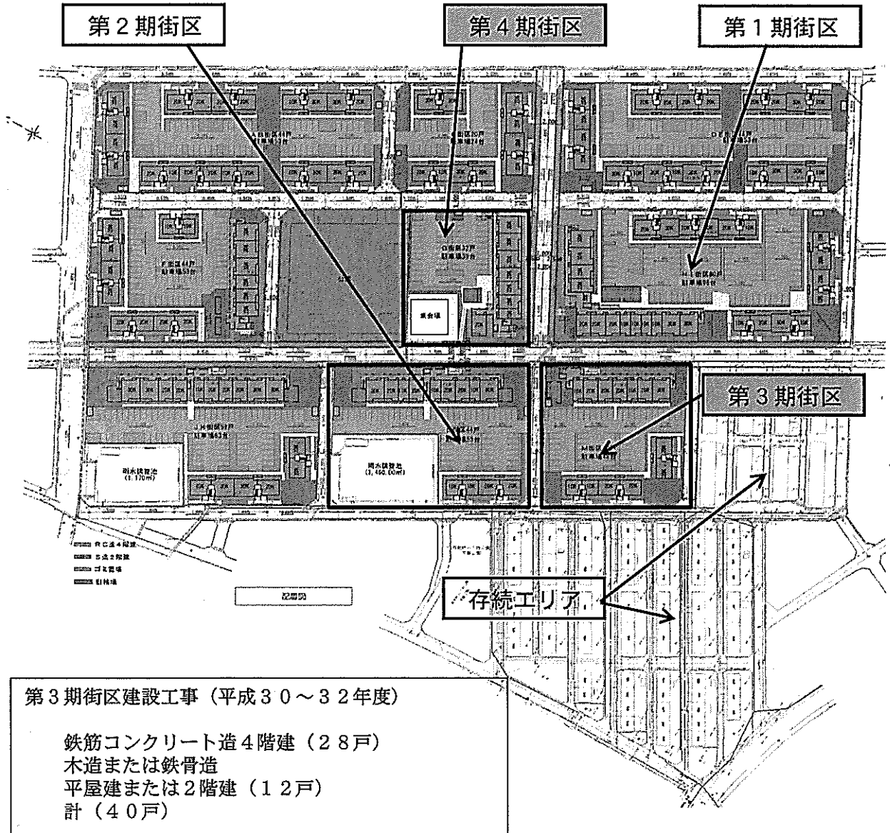
全体配置図
