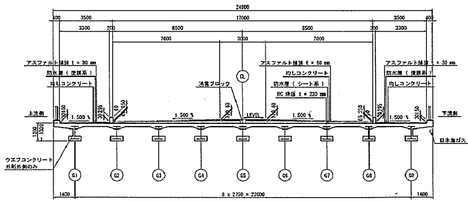
標準断面図
