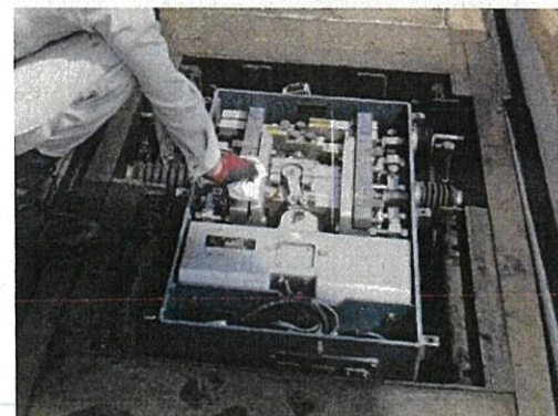
電気転てつ機内部
