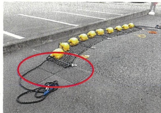
【すり抜け防止用フェンス】
