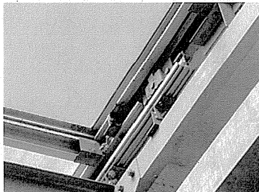
カーテンウォール取付け金物
