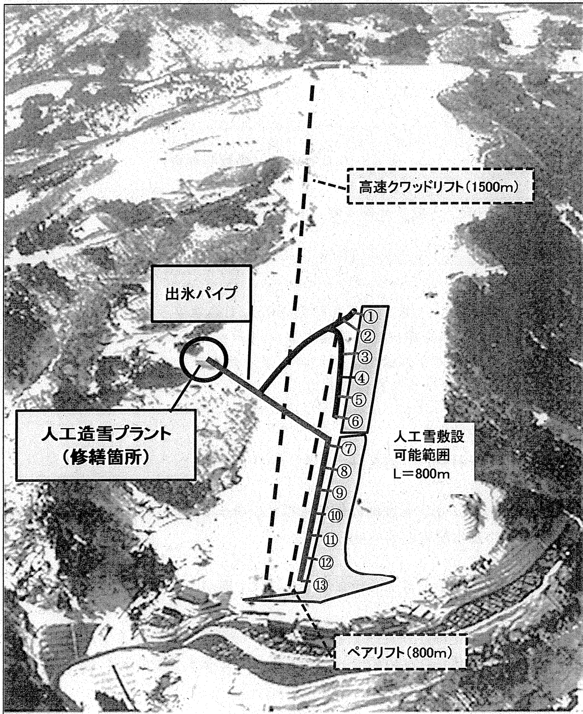
○ゲレンデ及び人工造雪プラント図
