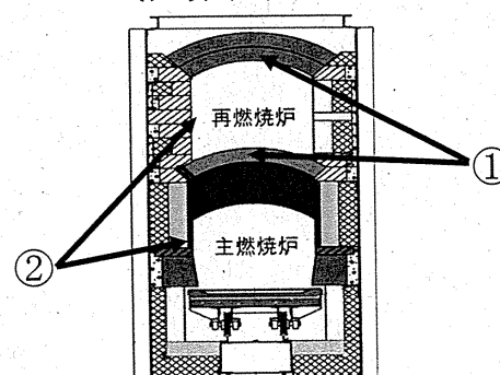
＜火葬炉断面図＞
