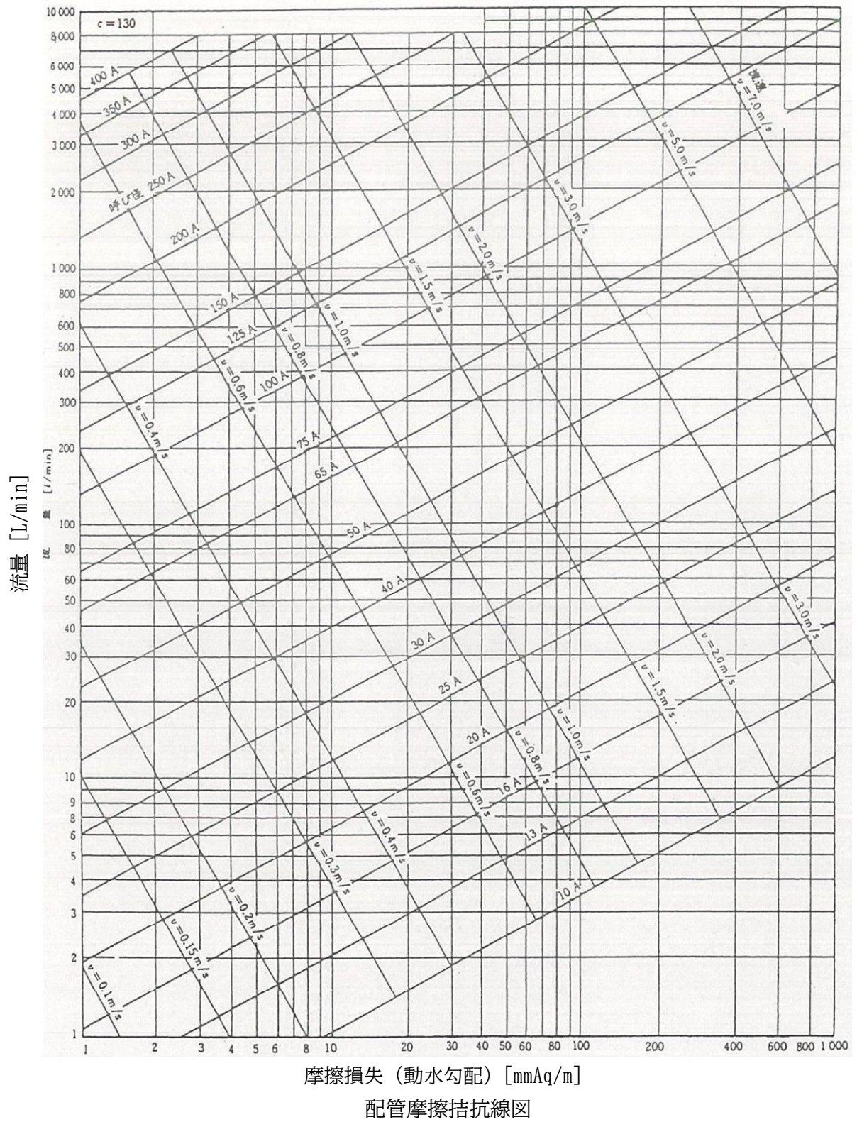
図2-2 ウィリアム・ヘーゼンの式による 硬質塩化ビニル管流量図
