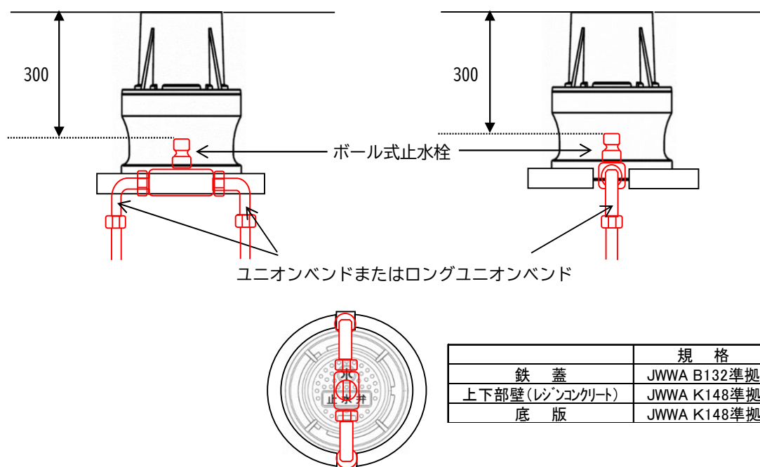
積上式 青銅製仕切弁用 (t-25 対応)
