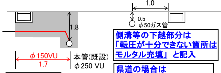
A-A' 断面
