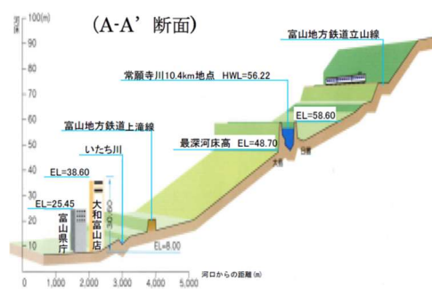
■常願寺川扇状地断面図
