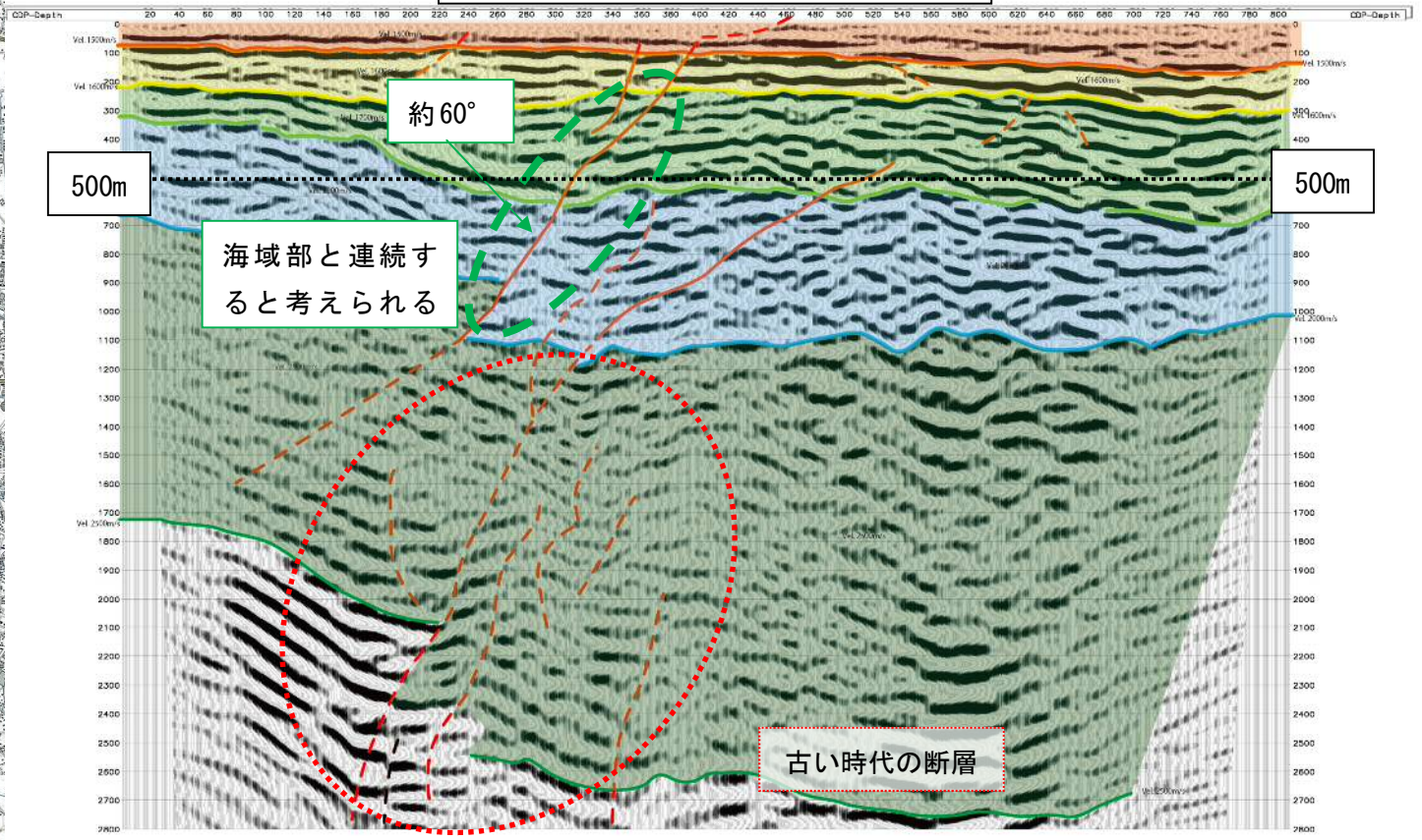
反射法探査断面図(海岸測線)及び解釈図
