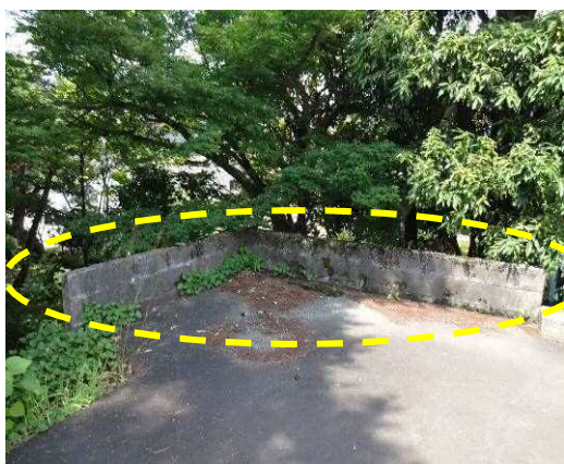
①塀の高さ 50 cm、長さ 5.5m 控壁なし
