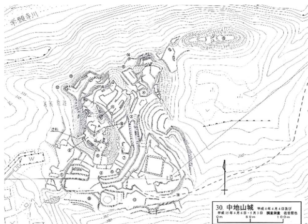
縄張り図
