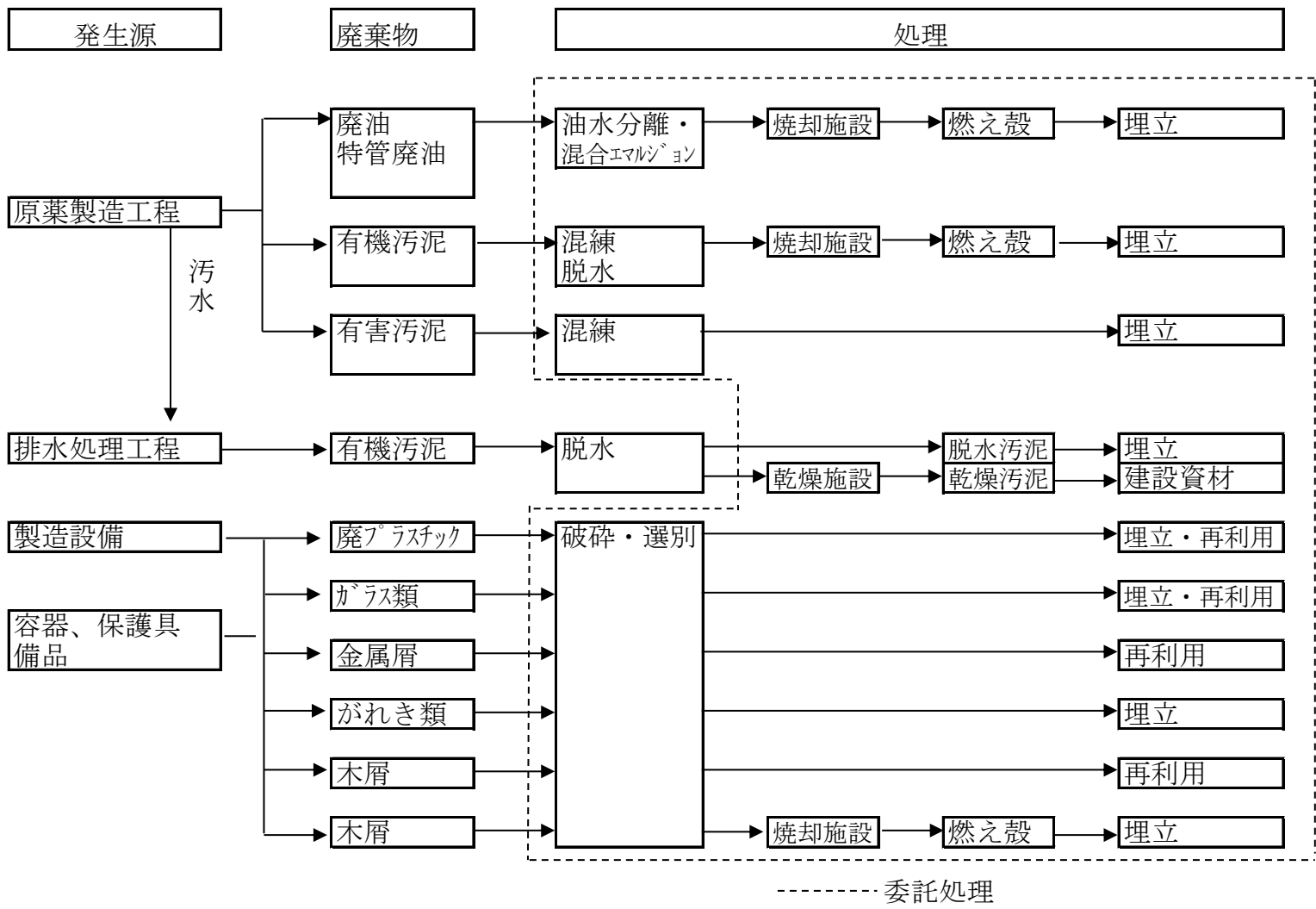
産業廃棄物の発生、委託処理フローシート
