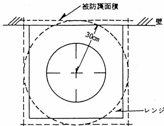
基準40-5図 レンジの被防護面積（コンロが1口の場合）
