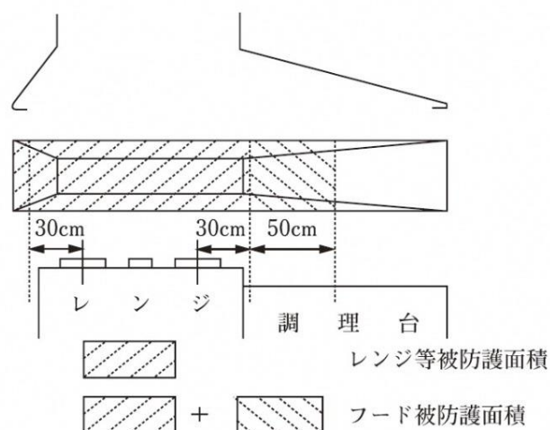
基準40-2図 レンジ又はフライヤーの被防護面積よりフードが大きい場合のフードの被防護面積（例）
