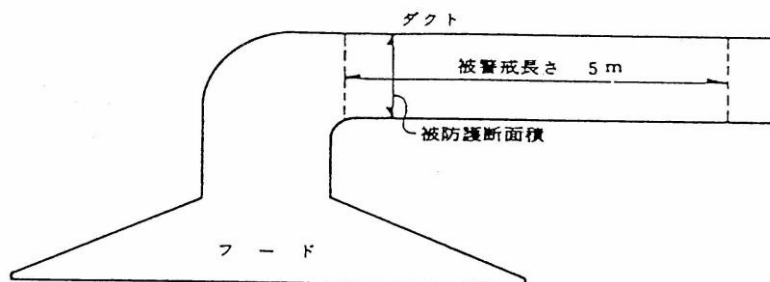
基準40-4図 ダクトの被警戒長さ及び被防護断面積
