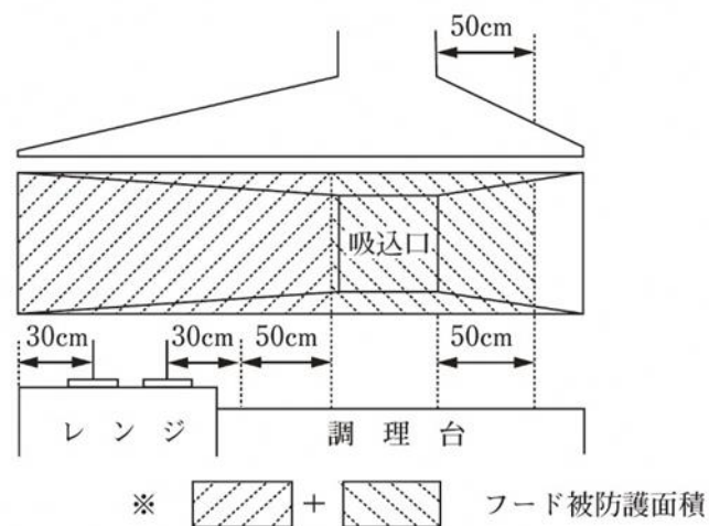
基準40-3図 ダクト吸入口がレンジの直上部以外の位置にある場合のフード被防護面積（例）
