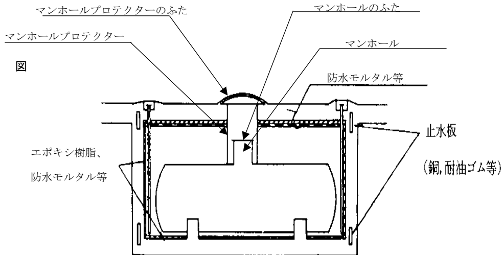
タンク室の防水措置の例
