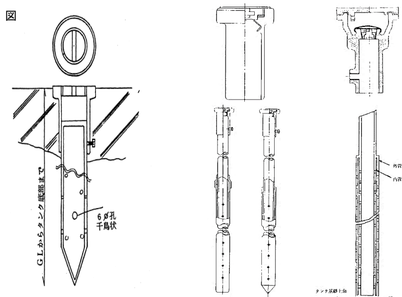
漏えい検査管の管体構造例
