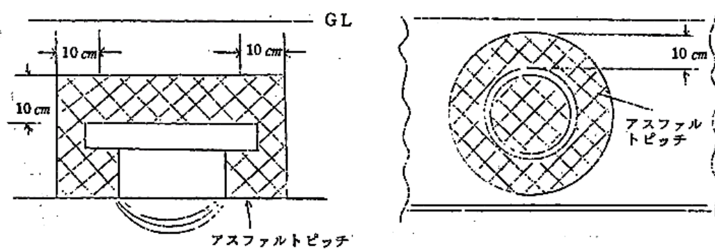
タンク室及びマンホールプロテクターを設けない地下貯蔵タンクのマンホールの保護方法例
