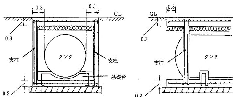
支柱により支える例（単位：m）
