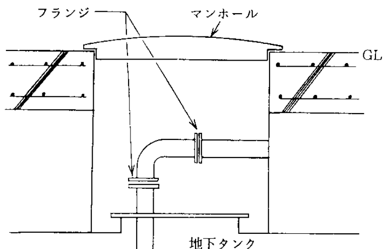
配管の接続例
