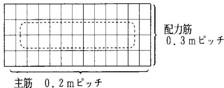
タンクふたの配筋例
