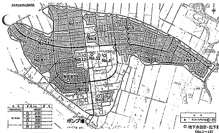
【上段】地下水位(単位:m) 【下段】沈下量(単位:mm)
