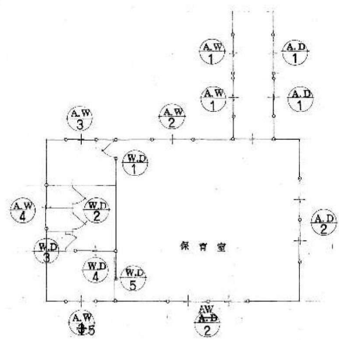
符号図 S=1/50
