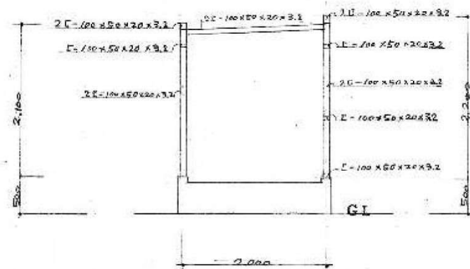
軸組図 S=1/50
