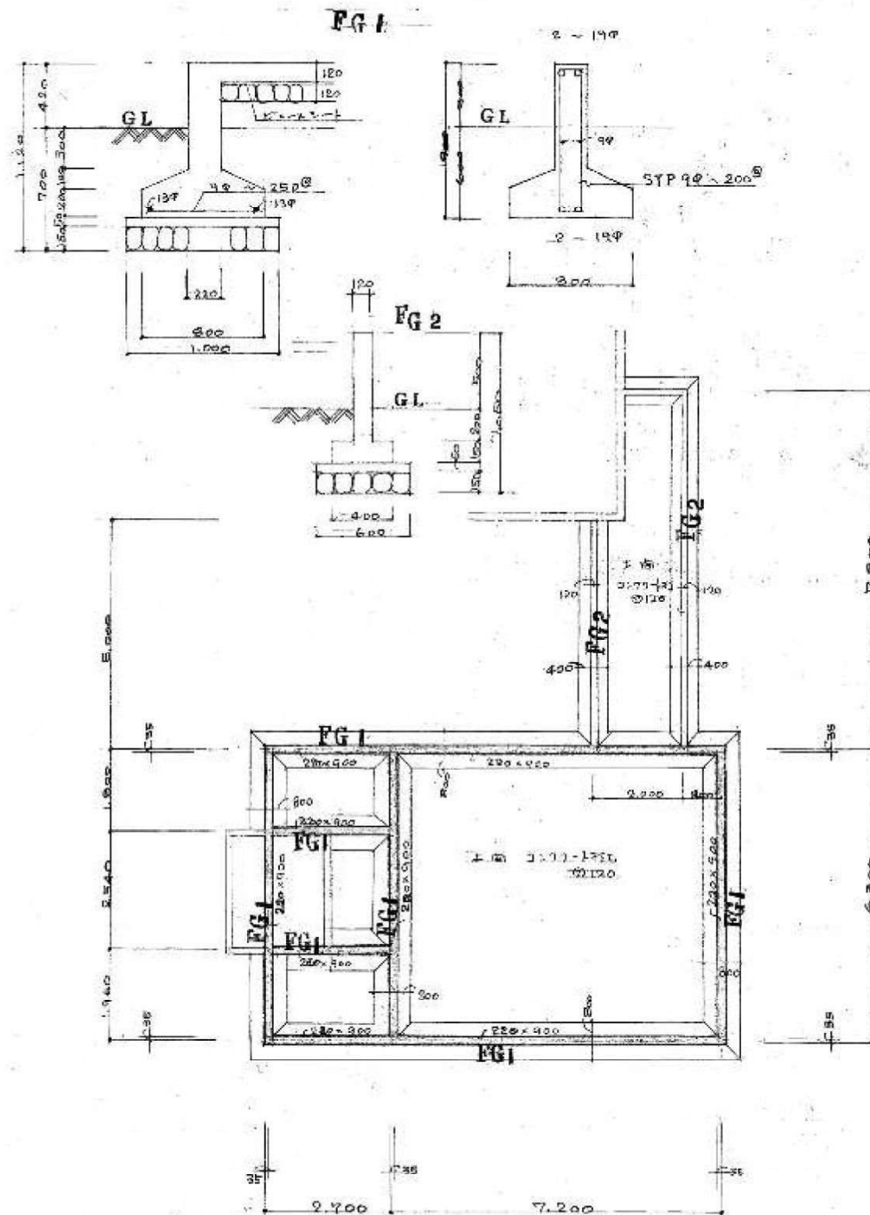
基礎伏図 S=1/100
