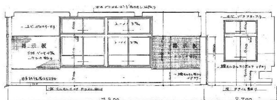
B-B 展開図 S=1/50
