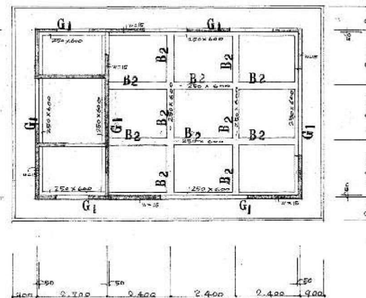
梁伏図 S=1/100
