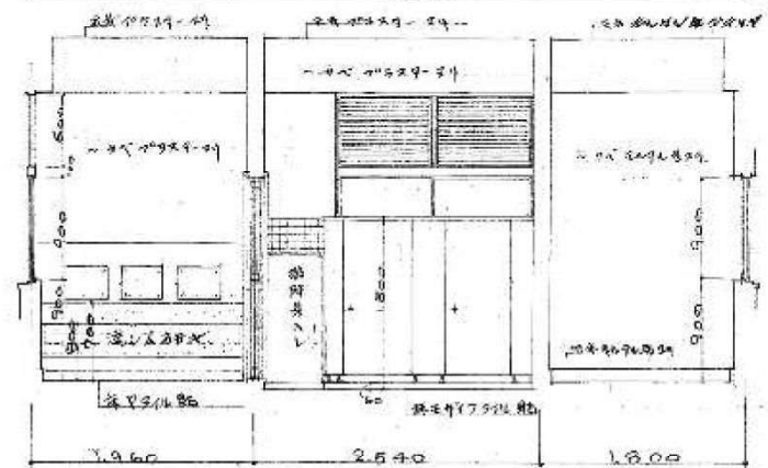
E-E 展開図 S=1/50
