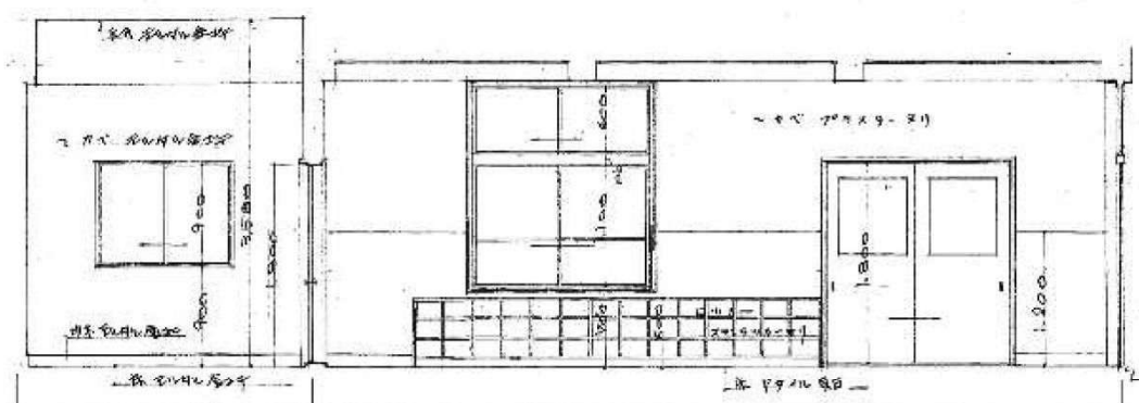
A-A 展開図 S=1/50
