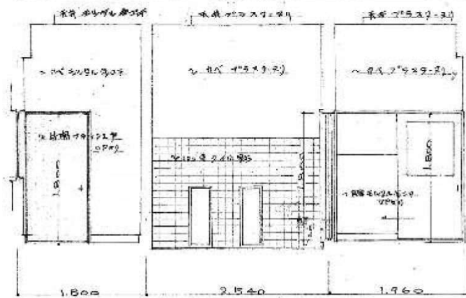
F-F 展開図 S=1/50
