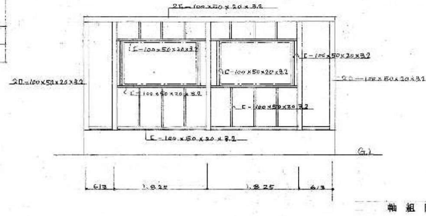
軸組図 S=1/50
